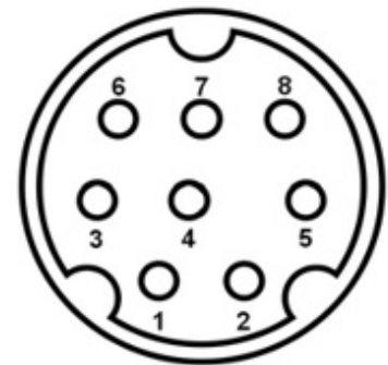
Mini DIN-8
