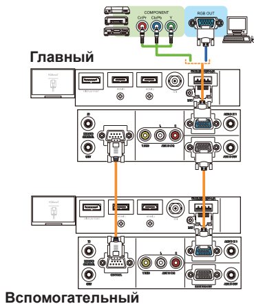
Пример подключения в интеллектуальный стек
