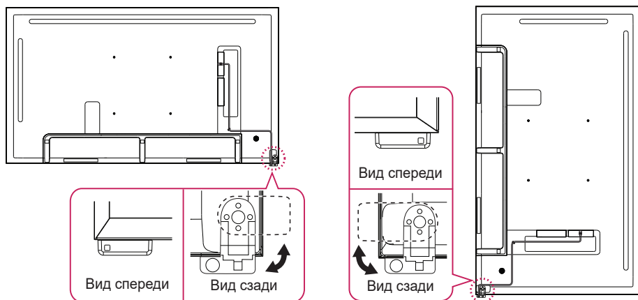
Монтаж в горизонтальном положении (по умолчанию)
